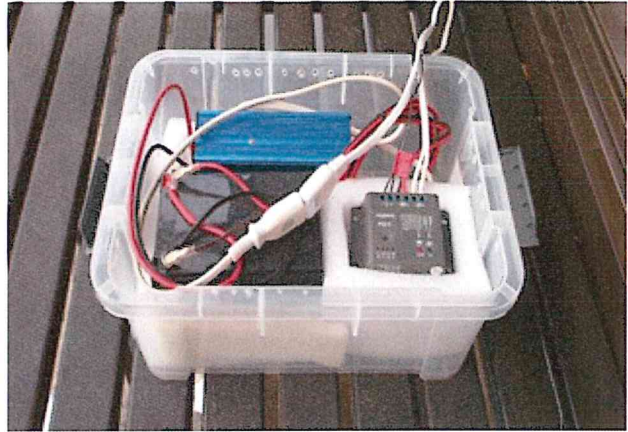
パネル以外の構成機器をボックスに収納 （Sさん宅 20W）
